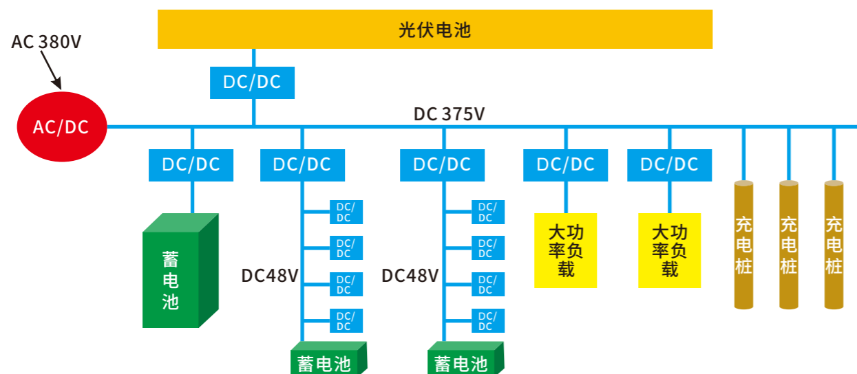
建筑“光储直柔”配电系统
