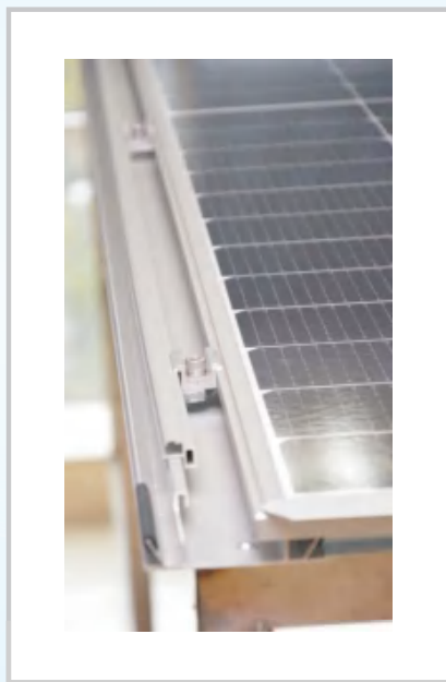
嵌入式防水组件
